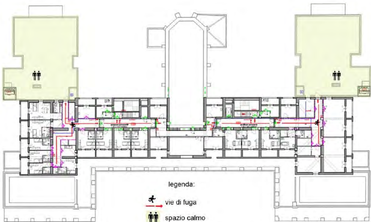
PROGETTO ANTINCENDIO – PIANO QUARTO
