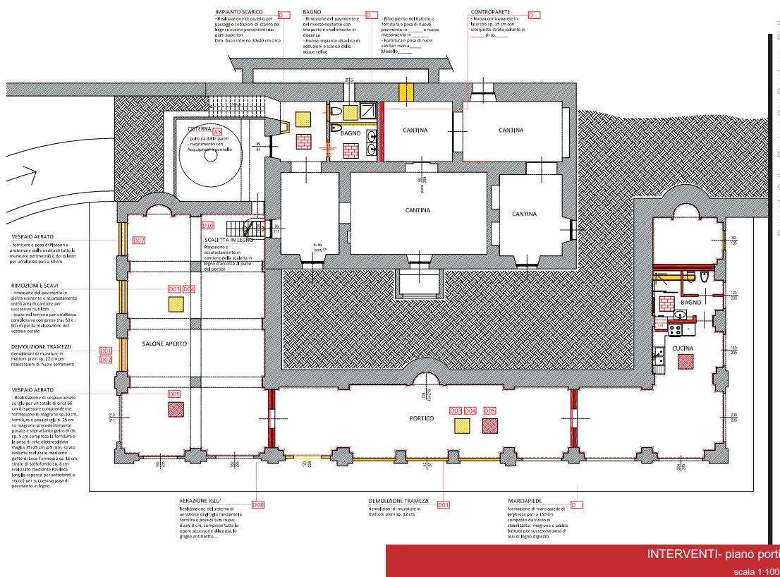
tavola del progetto esecutivo
